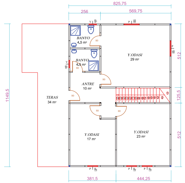
129 m2 PREFABRİK EV ÜST KAT PLANI
