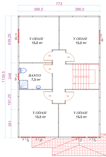
88 m2 ÜST KAT PLANI
