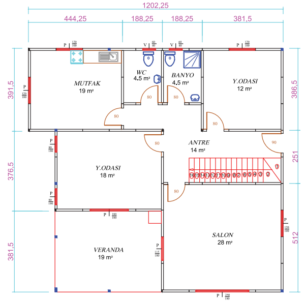
129 m2 PREFABRİK EV ZEMİN KAT PLANI
