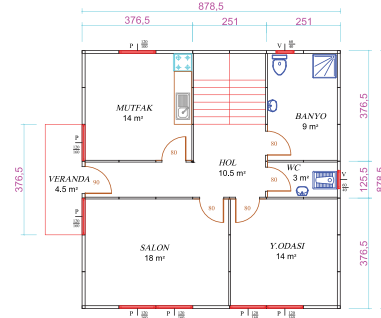
82 m2 DUBLEKS EV ZEMİN KAT PLANI
